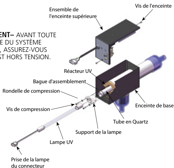
Figure 2: Vue éclatée du spa Solar Eclipse
